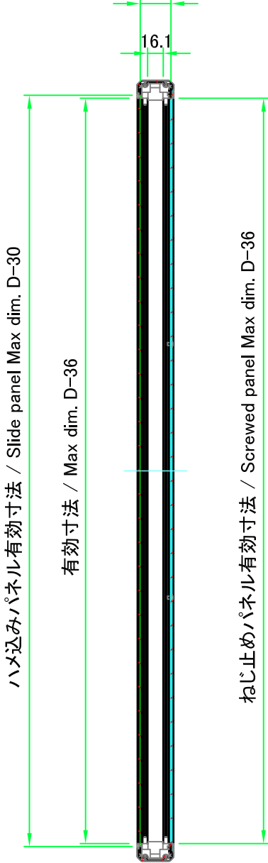
有効寸法 / Max dim. 31.5
